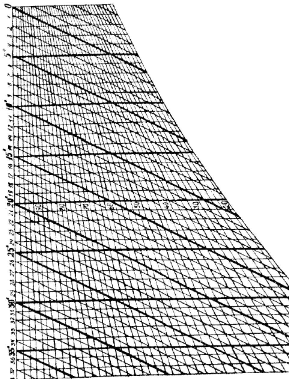
Рис. 3. Психрометрический график
